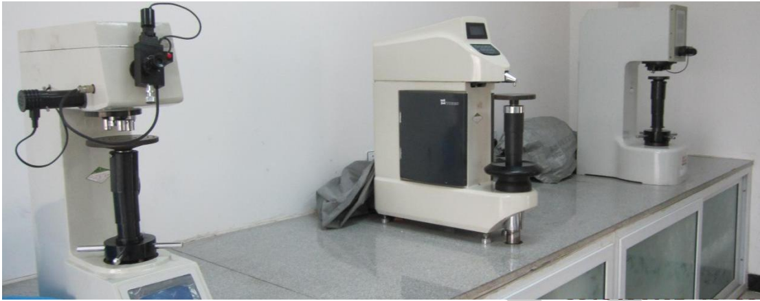
金属分析仪 (Hardness Test 硬度检测)
